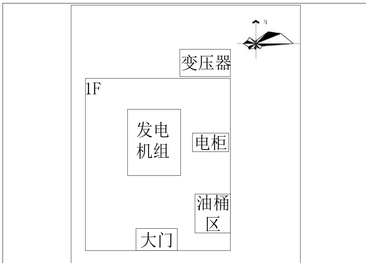
图4-3 项目总平面布置图（比例1:500）
