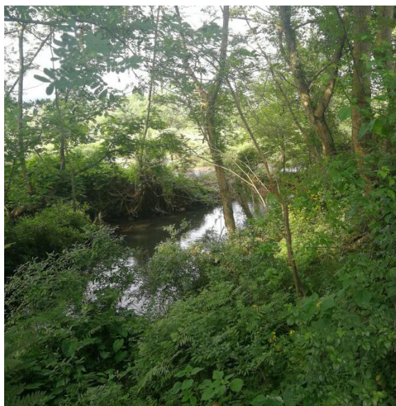
图5-2 减水区生境
