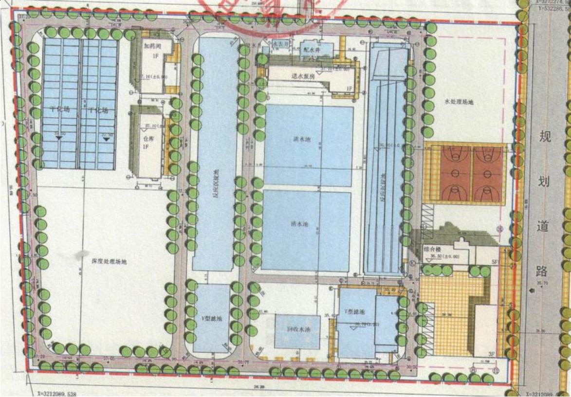
图 2.2 项目建筑物平面布置
